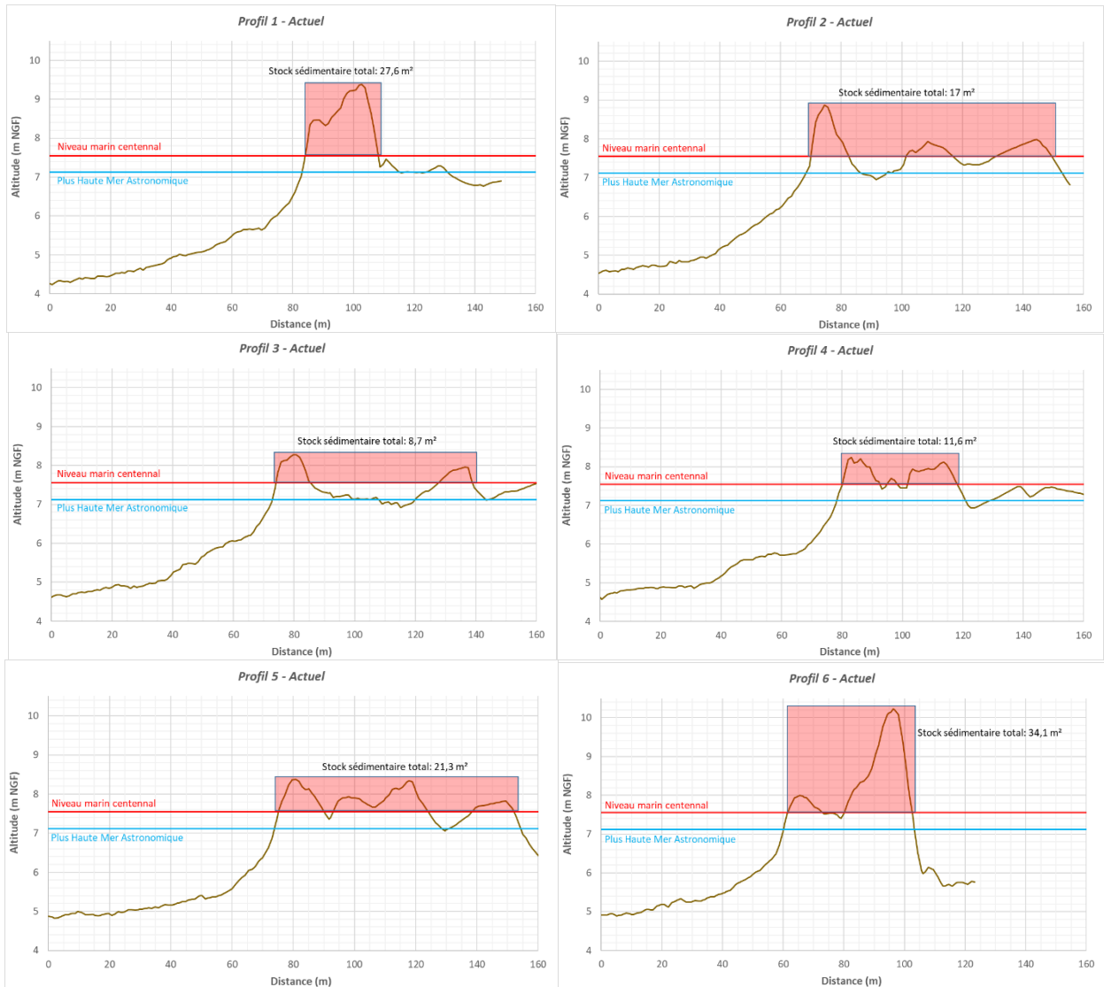
Illustration 49 – Vue des 6 profils topographiques analysés sur le cordon dunaire de la Roche Morin (d'après les données du RGE Alti du début des années 2010) et estimation des stocks sédimentaires totaux.
