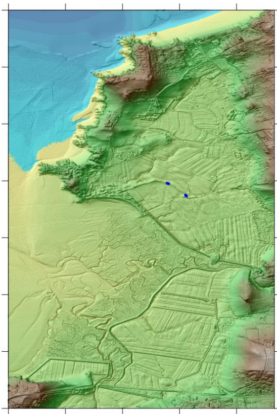
Illustration 74 – Scénario d'aménagement CA1 : Comblement des 2 brèches dans la digue des Moines à Lancieux (en bleu).
