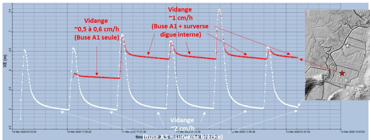
Illustration 65 – Evolution des niveaux d'eau dans la partie principale du polder de Ploubalay (en blanc) et dans le compartiment Sud du polder (en rouge) pendant la simulation du scénario B_2020, avec estimation des vitesses de vidange associées.
