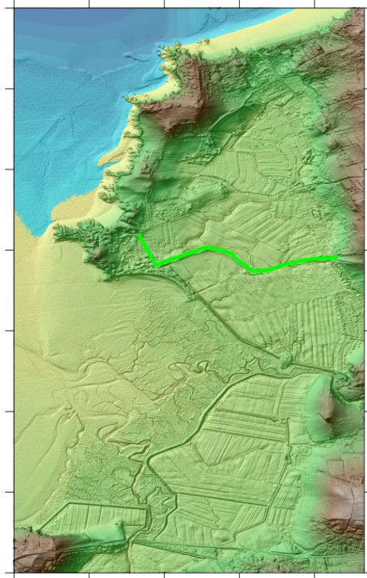
Illustration 77 – Scénario d’aménagement CA4 : Construction d’une digue rétro-littorale suivant la digue des Moines à Lancieux (en vert).
