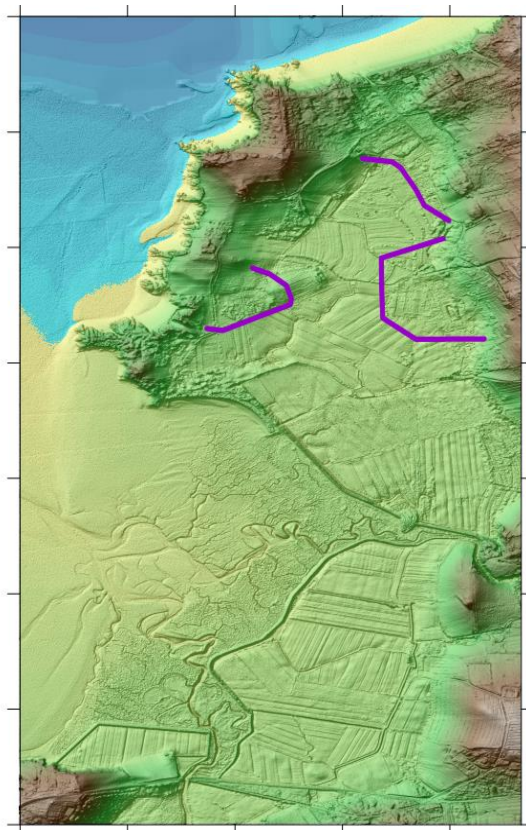
Illustration 78 – Scénario d’aménagement CA5 : Construction de 3 digues rétro-littorales au plus près des enjeux à Lancieux (en violet).
