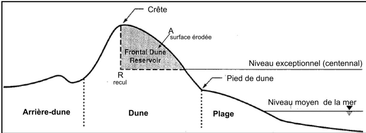
Illustration 47 - Représentation du calcul du volume du stock maximal mobilisable par un événement caractérisé par un niveau d'eau centennal, valeur limite avant disparition de la dune (Source : FEMA, 1995).
