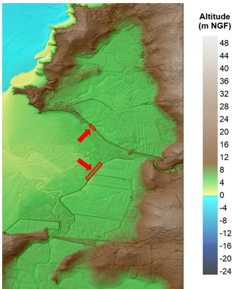
Illustration 60 – Aperçu des brèches envisagées dans les digues de la Roche et des Marais-Neufs et de leurs localisations.
