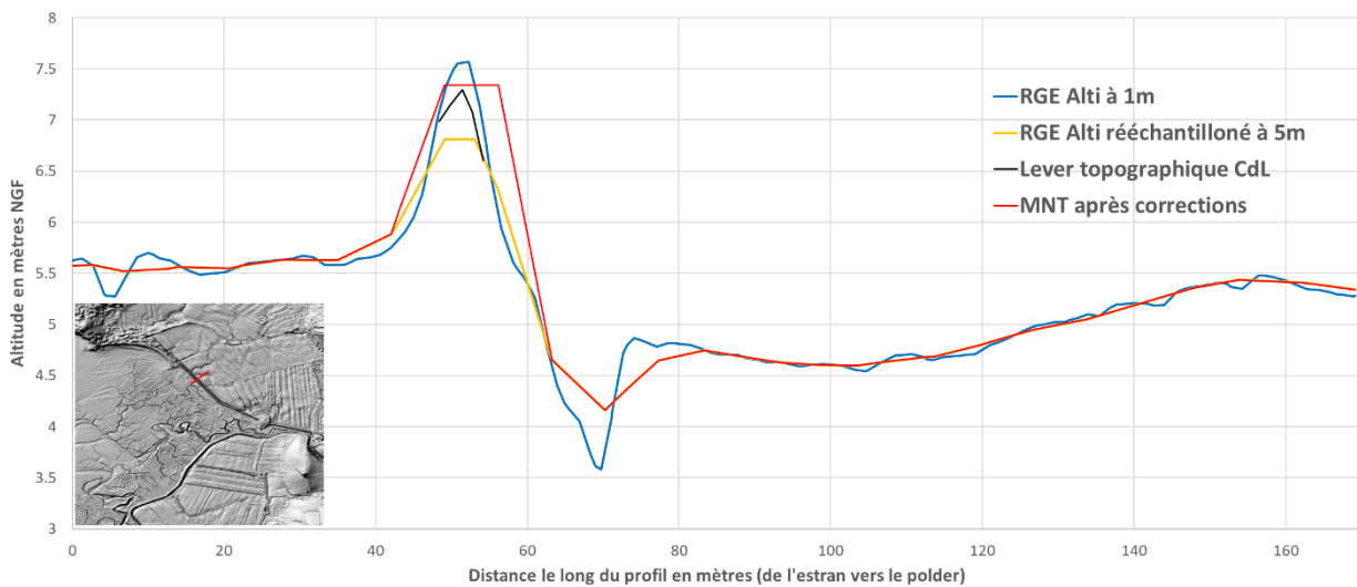
Illustration 54 – Aperçu des corrections apportées aux éléments structurants à travers l'exemple d'un profil sur la digue de la Roche.
