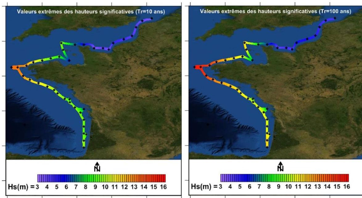
Illustration 34 – Hauteurs significatives des vagues au large pour des périodes de retour de 10 ans (à gauche) et 100 ans (à droite) estimées à partir de la base BoBWA (Charles et al., 2012) sur la période 1958-2001 à pas de temps 6 heures (Bulteau et al., 2013).
