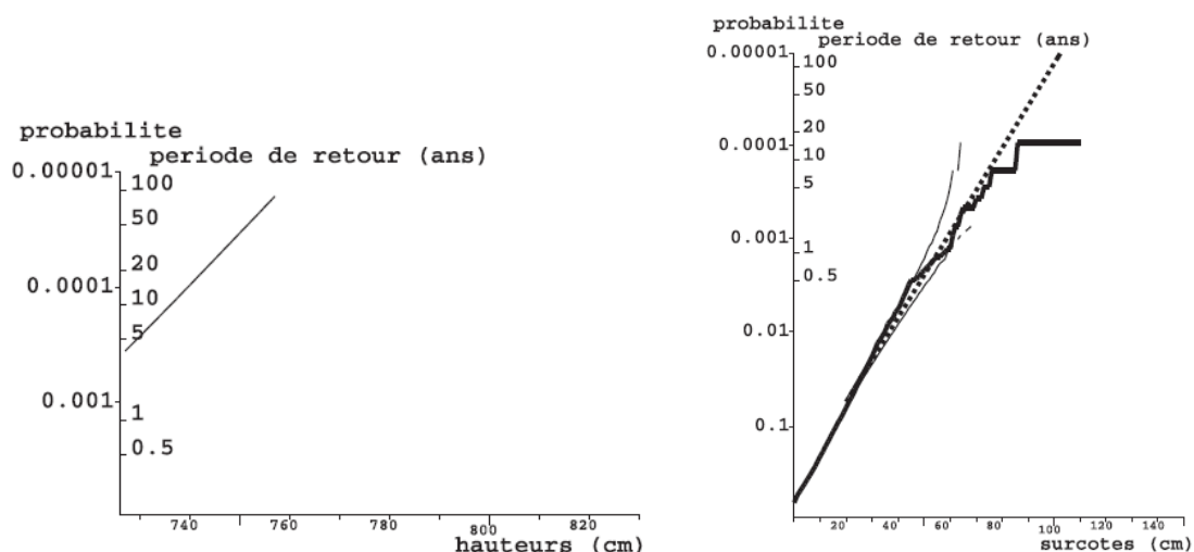
Illustration 31 - Période de retour des hauteurs/niveaux marins extrêmes de pleine mer (à gauche) et des surcotes (à droite) à Saint-Malo (extrait de SHOM-CEREMA, 2012).
