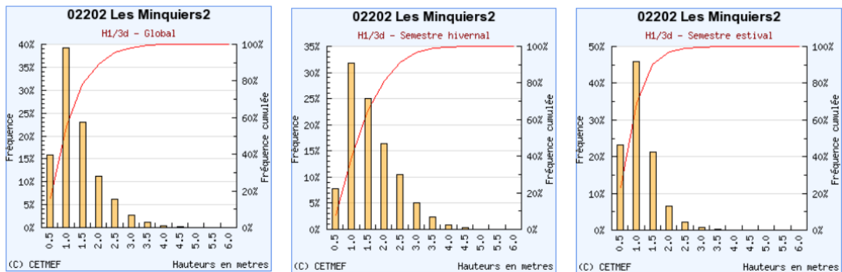
Illustration 37 - Histogramme représentant la fréquence des hauteurs significatives des houles mesurées à la bouée 02202 – Minquiers 2, sur la période 1997 – 2009, en considérant toute la période à gauche, puis la période hivernale au centre et la période estivale à droite ( http://candhis.cetmef.developpement-durable.gouv.fr ).
