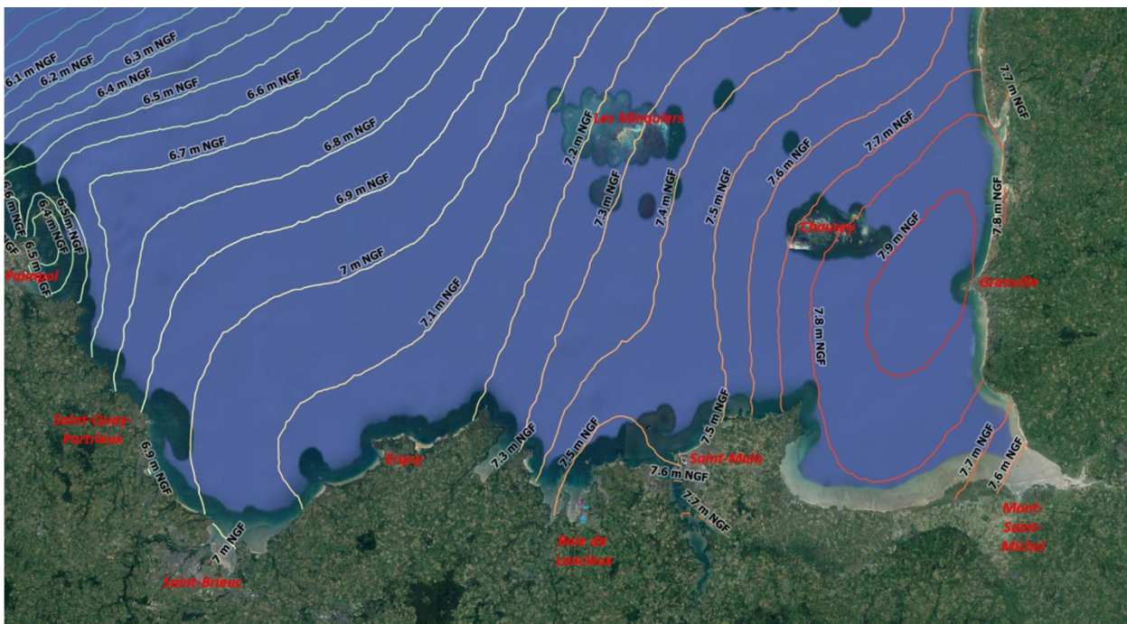
Illustration 33 - Niveaux centennaux de pleine mer dans le golfe normano-breton (d'après SHOM-CEREMA, 2012).
