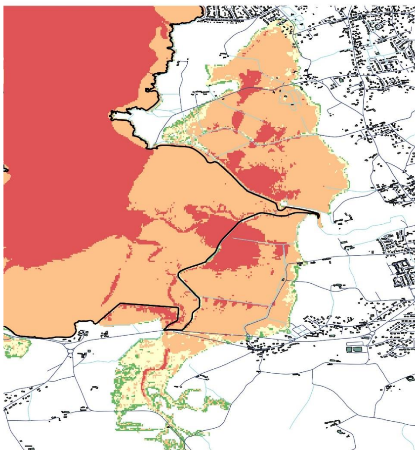
Illustration 69 – Carte d'aléa pour le scénario centennial B_2100 (Digue de la Roche intacte, brèche dans la digue des Marais-Neufs, échéance post 2050).
