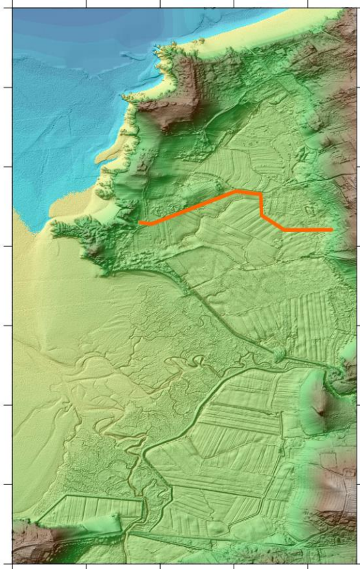
Illustration 76 – Scénario d’aménagement CA3 : Construction d’une digue rétro-littorale suivant la rue des Bénédictins à Lancieux (en orange).
