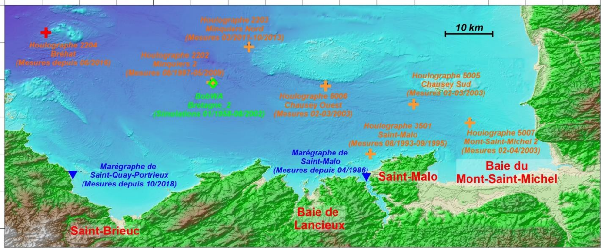
Illustration 29 – Localisation des mesures disponibles autour du site de la Baie de Lancierx (marégraphes en bleu, houlographes en orange, point d'analyse statistique des vagues issu de l'atlas numérique d'états de mer BoBWA en vert).
