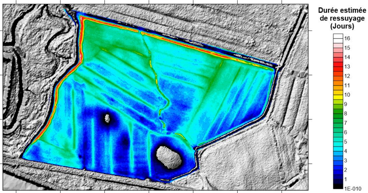
Illustration 66 – Estimation des durées de ressuyage dans le compartiment Sud du polder de Ploubalay en partant d'un remplissage au niveau marin centennal.
