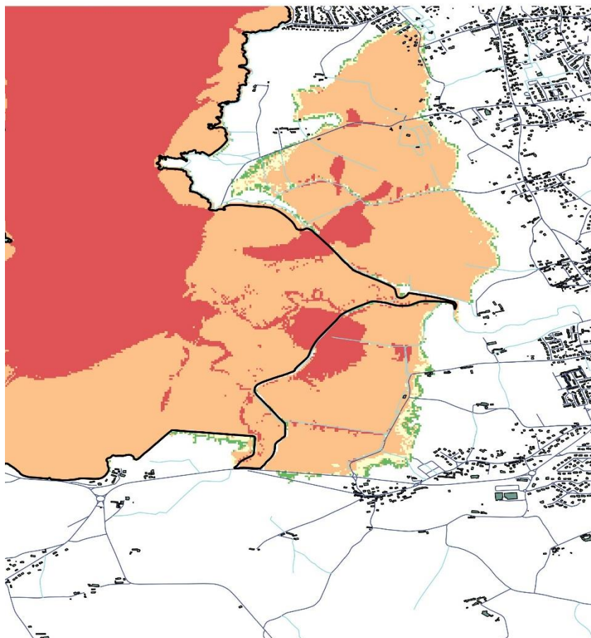
Illustration 70 – Carte d'aléa pour le scénario centennal C_2020 (Brèches dans les digues de la Roche et des Marais-Neufs, échéance actuelle).
