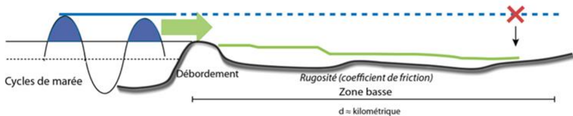
Illustration 50 - Schéma de principe de la méthodologie employée pour la propagation de la submersion marine : le niveau marin de référence (bleu continu) n'est pas simplement projeté sur la topographie (bleu pointillé) mais bien propagé suivant une dynamique de submersion (vert).
