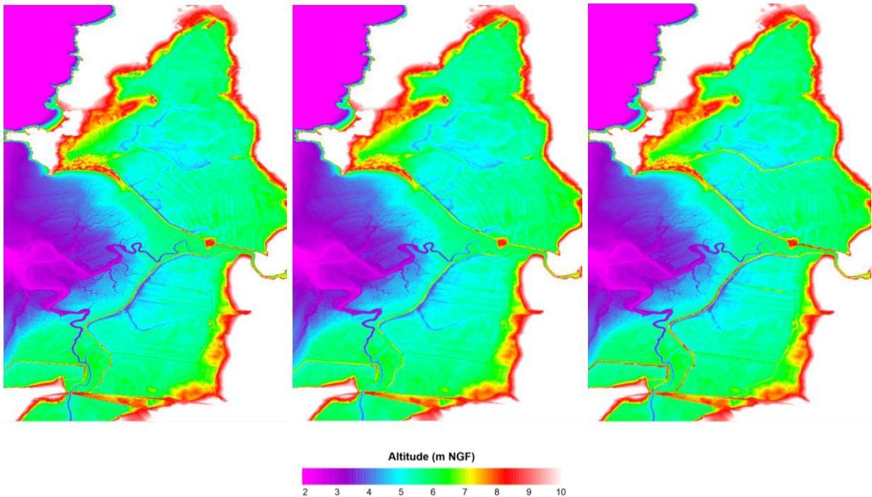
Illustration 55 – Construction du MNT : A gauche : RGE Alti à 1 m ; Au centre : après ré-échantillonnage à 5 m ; A droite : Après correction des éléments structuraux.
