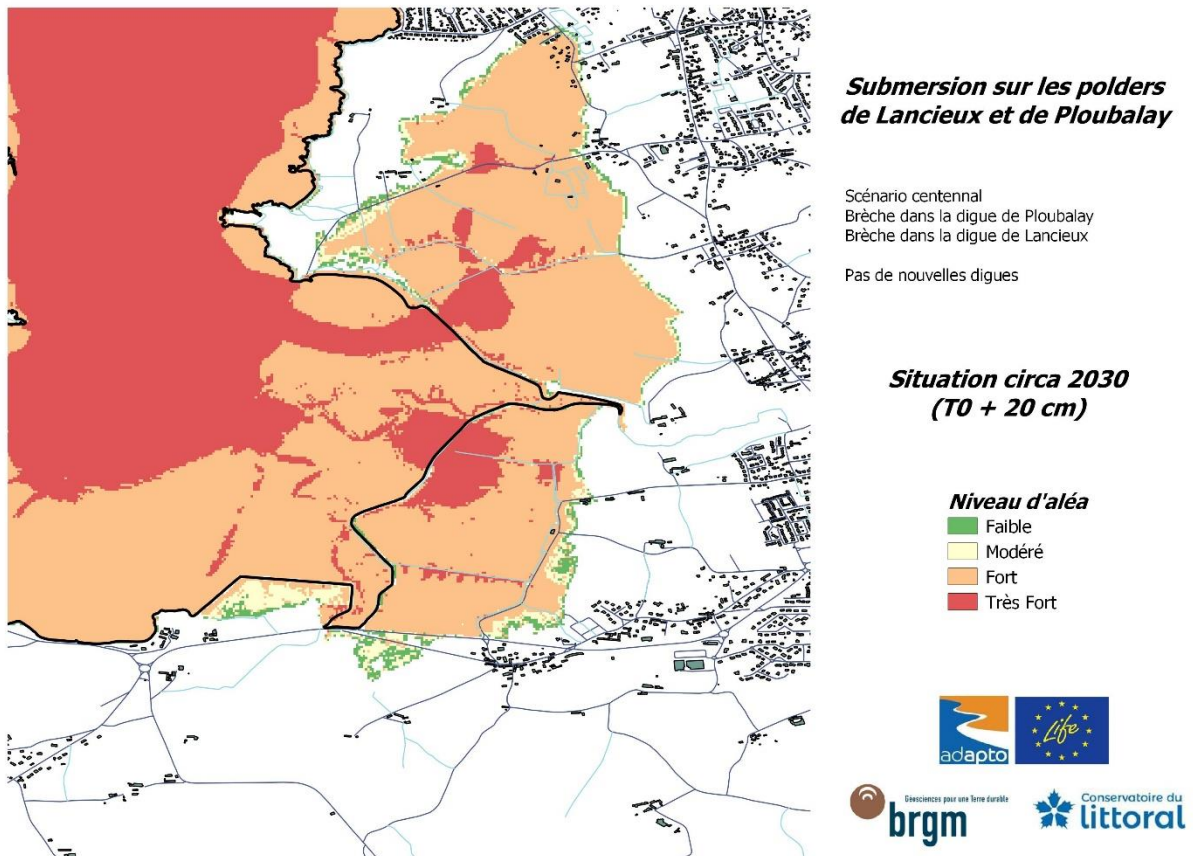
Illustration 71 – Carte d'aléa pour le scénario centennial C_2030 (brèche dans la digue de la Roche intacte, brèche dans la digue des Marais-Neufs, échéance circa 2030).
