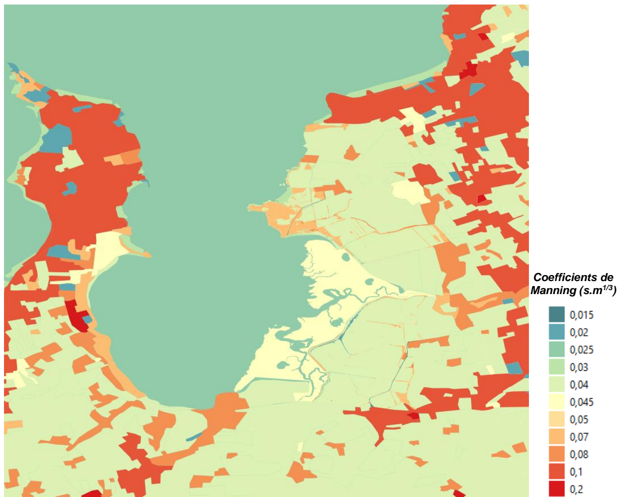
Illustration 56 – Carte des coefficients de Manning (frottements au sol) établie sur la base des données d'occupation des sols.
