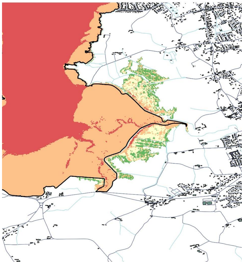
Illustration 63 – Carte d'aléa pour le scénario centennal A_2020 (Digues de la Roche et des Marais-Neufs intactes, échéance actuelle).
