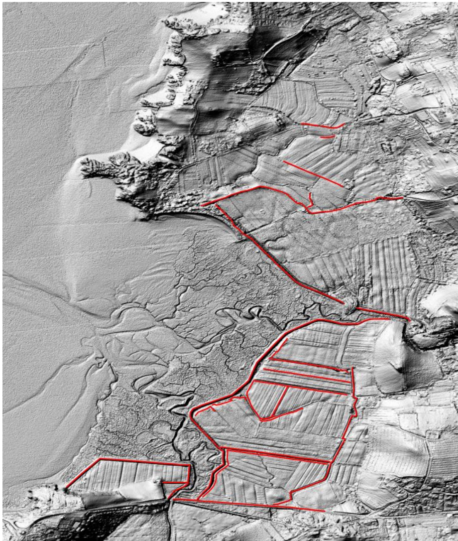
Illustration 53 – Identification des éléments structurants susceptibles d'avoir été « gommés » lors de l'élaboration du MNT topo-bathymétrique
