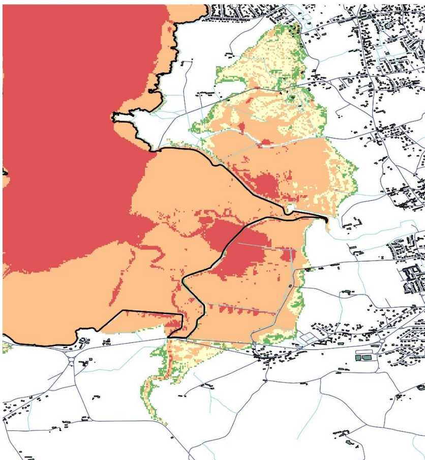
Illustration 68 – Carte d'aléa pour le scénario centennial B_2050 (Digue de la Roche intacte, brèche dans la digue des Marais-Neufs, échéance circa 2050).
