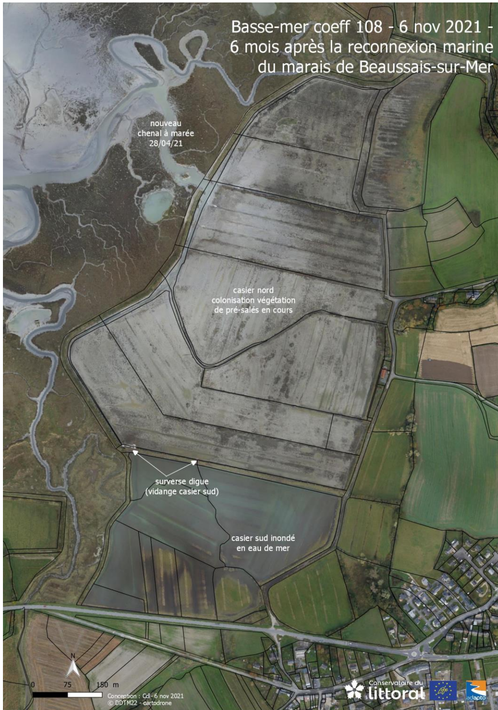
Illustration 19 – Vue aérienne en orthomosaïque du polder de Ploubalay le 06/11/2021, montrant la brèche, le chenal et les zones submergées (conception Conservatoire du littoral d’après des images acquises par Cartodrone pour le compte de la DDTM des Côtes d’Armor).
