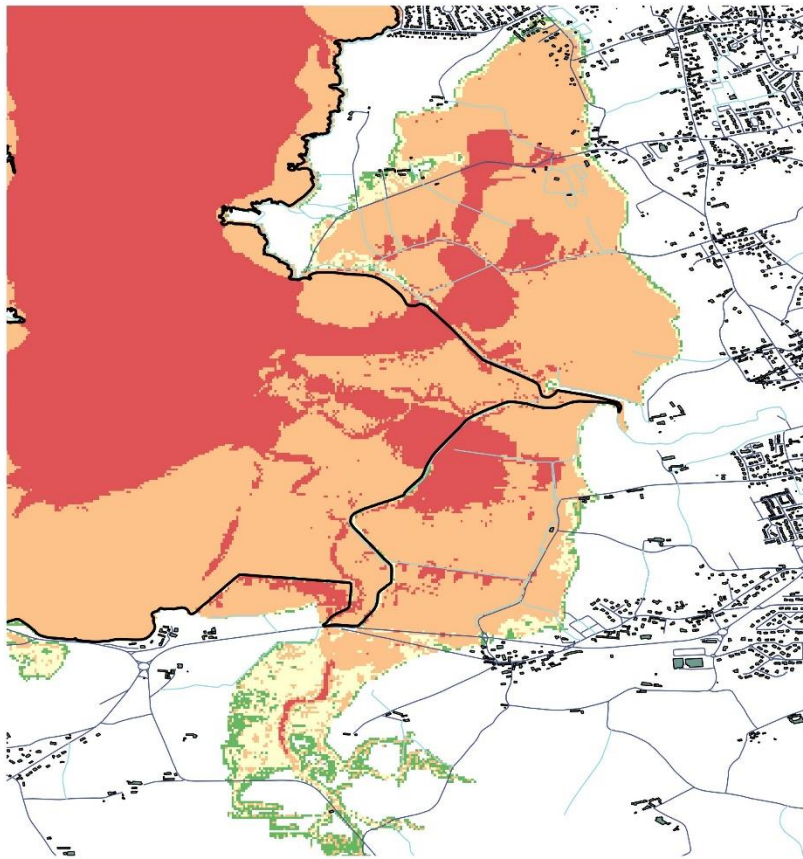
Illustration 73 – Carte d'aléa pour le scénario centennal C_2100 (brèche dans la digue de la Roche intacte, brèche dans la digue des Marais-Neufs, échéance post 2050).
