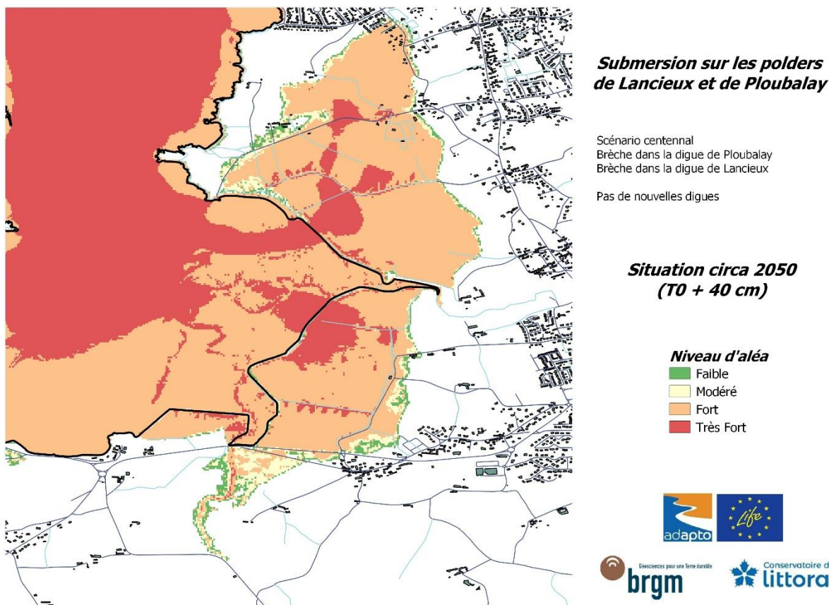
Illustration 72 – Carte d'aléa pour le scénario centennial C_2050 (brèche dans la digue de la Roche intacte, brèche dans la digue des Marais-Neufs, échéance circa 2050).
