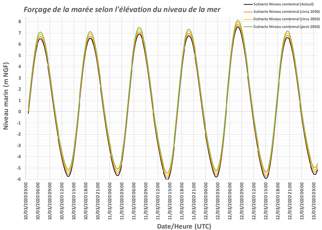
Illustration 59 – Signal de forçage de la marée utilisé pour les différentes échéances considérées.
