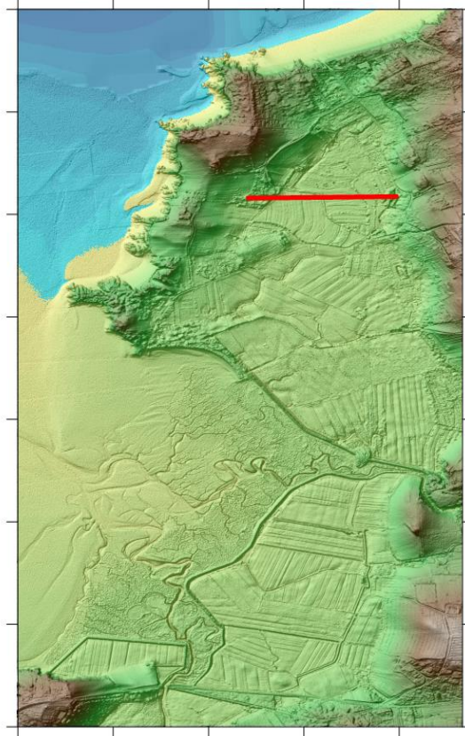
Illustration 75 – Scénario d'aménagement CA2 : Construction d'une digue rétro-littorale protégeant l'extrémité Nord du polder de Lancieux (en rouge).
