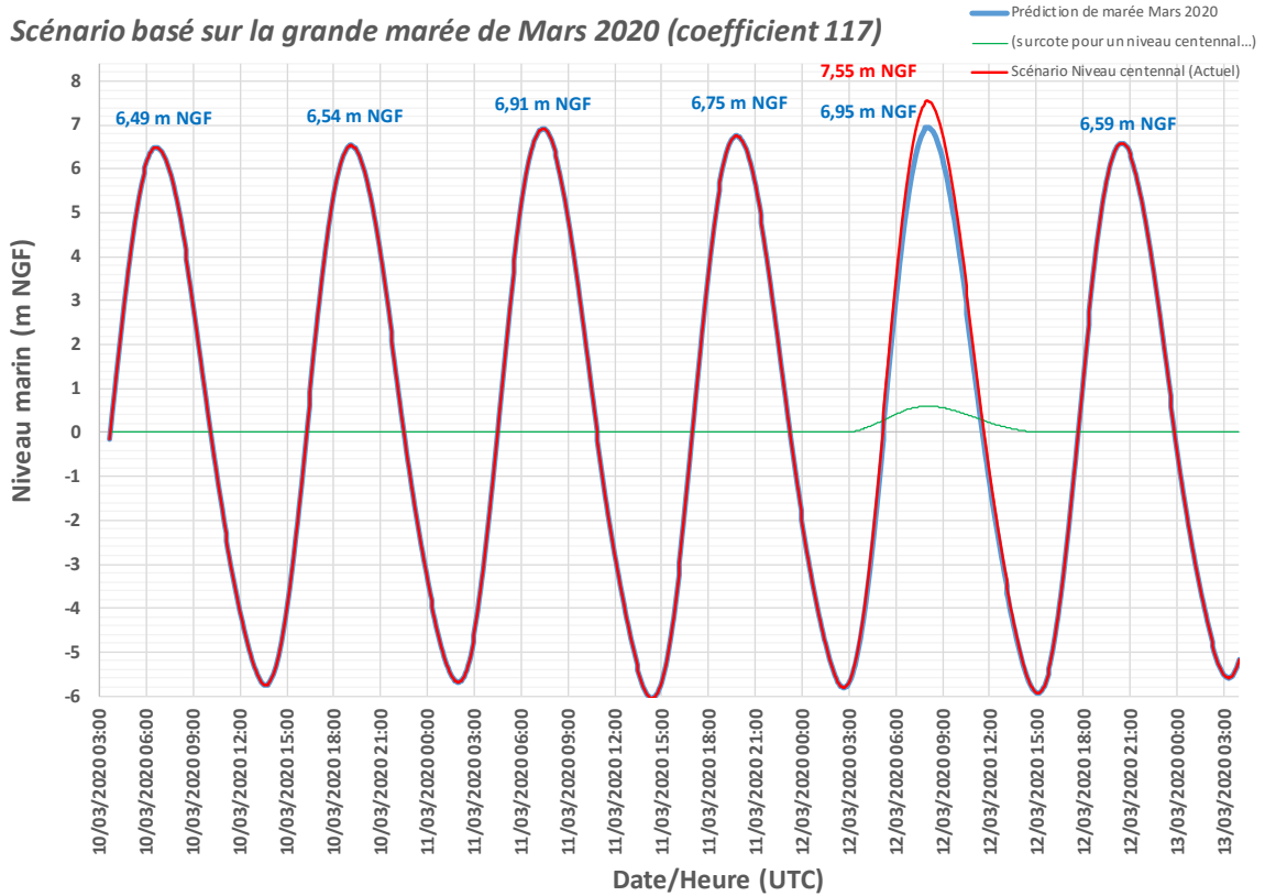
Illustration 58 – Grande marée du 10 au 13 Mars 2020 (coefficients 111 à 117) : prédiction de marée (en bleu), scénario centennial (en rouge) et surcote correspondante (en vert).
