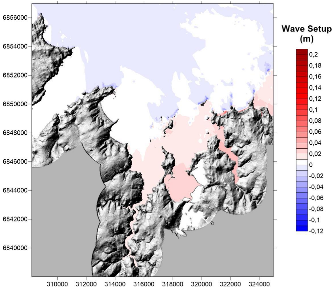
Illustration 40 - Exemple de simulation de la propagation des vagues depuis le large jusqu'à l'intérieur de la Baie de Lancieux : Aperçu du wave setup (surcote générée par le déferlement des vagues) configuration stationnaire avec un niveau marin correspondant aux Plus Hautes Mers Astronomiques et à des vagues au large du type de celles de la tempête Éléonor le 03/01/2018 : H_s = 3,75 m et T_p = 12 s.
