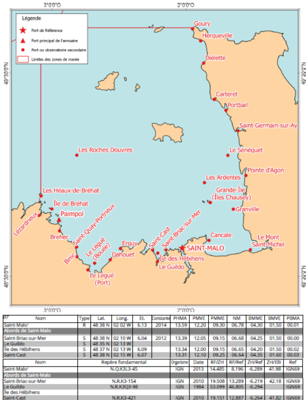
Illustration 30 – Rattachement des ports du golfe normano-breton, dont le port de référence est celui de Saint-Malo, et références altimétriques maritimes sur la Côte d’Emeraude (Source : Shom, 2019).
