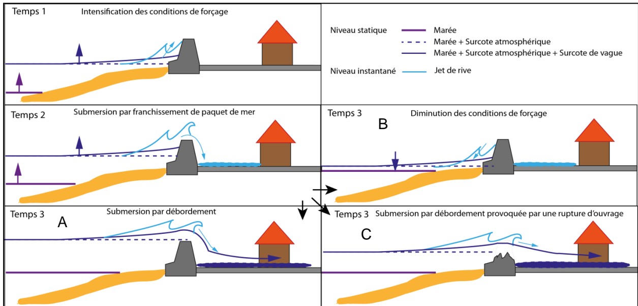
Illustration 23 - Exemple de chronologies possibles en cas de submersion marine (franchissement par paquets de mer / dégradation des ouvrages / débordement, ©BRGM).
