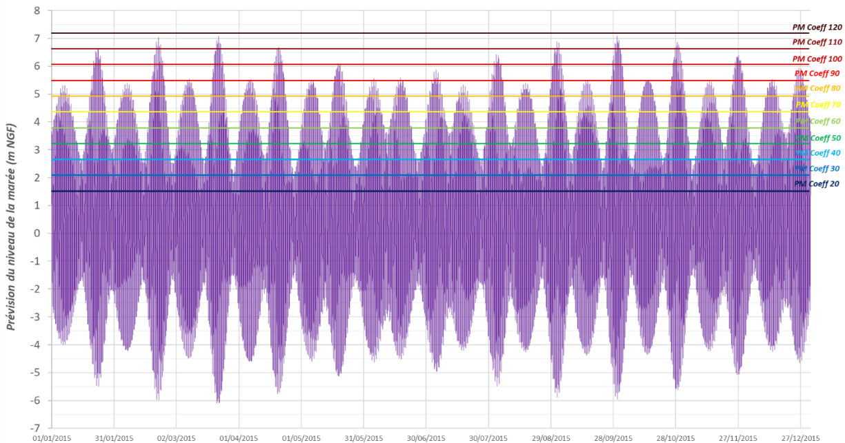
Illustration 41 – Aperçu des niveaux marins prévus aux Hébihens pour l'année 2015 (les droites horizontales correspondent aux niveaux moyens caractéristiques des pleines mers selon les coefficients déterminés au paragraphe 3.1).
