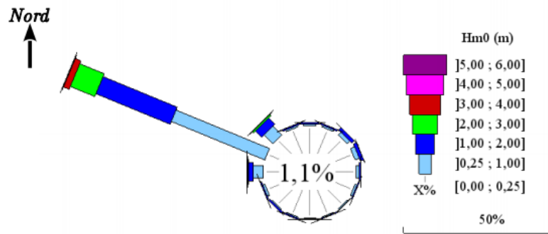
Illustration 36 - Rose des houles mesurées à la bouée 02202 – Minquiers 2 -, sur la période 1997– 2009 ( http://candhis.cetmef.developpement-durable.gouv.fr ).
