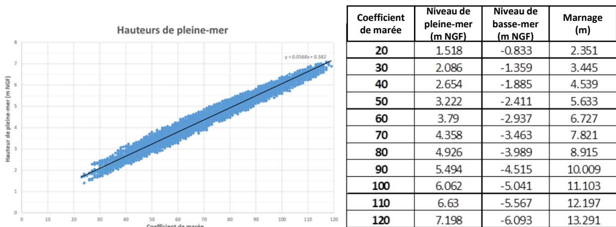
Illustration 38 – Prédiction des niveaux de pleine-mer aux Hébihens en fonction des coefficients de marée sur la période 2006-2015 (à gauche) et sélection de niveaux de pleine-mer et de basse-mer et de marnages représentatifs par décile de coefficients de marée (à droite).
