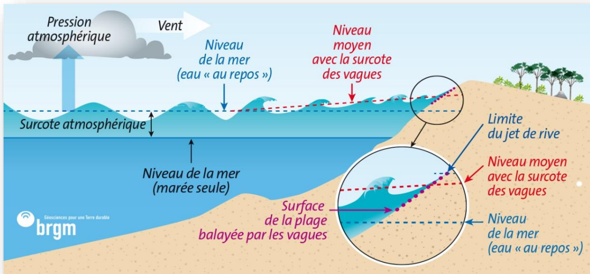
Illustration 22 - Schéma des différentes contributions au niveau du plan d'eau lors d'une tempête (surcotes) jusqu'au rivage.
