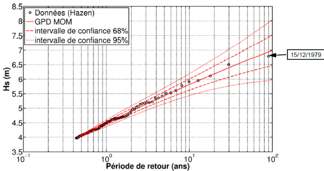
Illustration 35 – Analyse statistique des vagues au point BoBWA Bretagne_2 (Bulteau et al., 2013).
